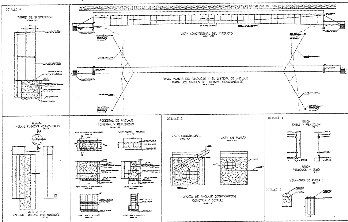
Ilustración 1 Detalle viaducto de 80 metros. Fuente: Archivos del proyecto
