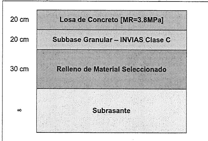
Ilustración 1 Detalle de la estructura de pavimento a construir Fuente: Archivos del proyecto – Diseño de Pavimento Rígido
