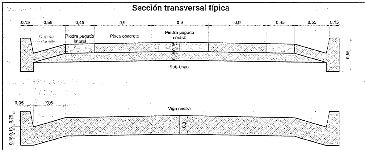
Ilustración 2 Detalle de la estructura a construir Fuente: Archivos del proyecto – Diseño de Pavimento
