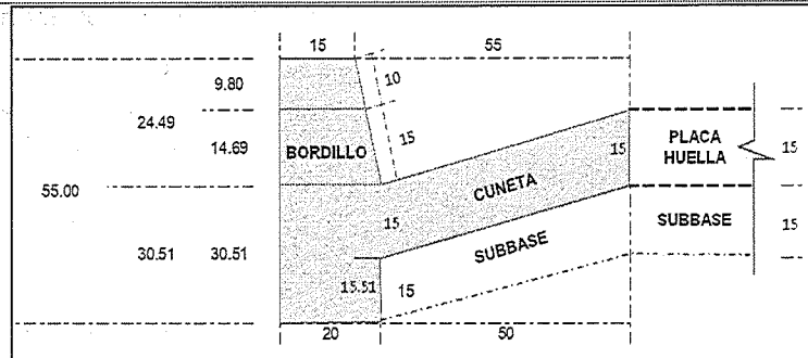
Ilustración 1 Detalle de las cunetas y bordillos Fuente: Archivos del proyecto – Memorias del cálculo
