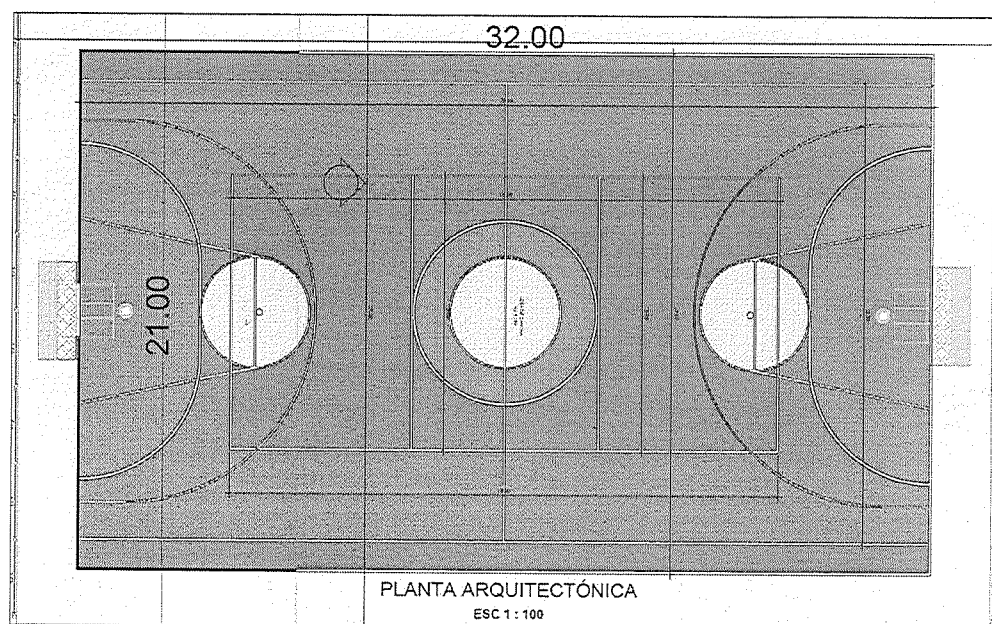
Ilustración 2 Detalle arquitectónico cancha.
