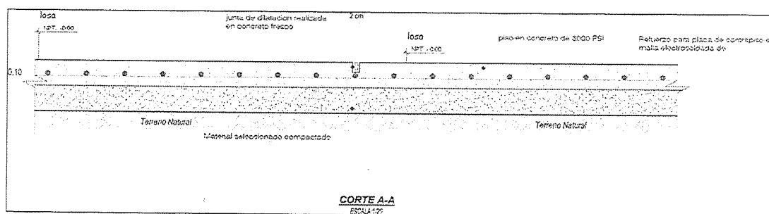
Ilustración 3 Detalle acero de refuerzo placa a construir.
