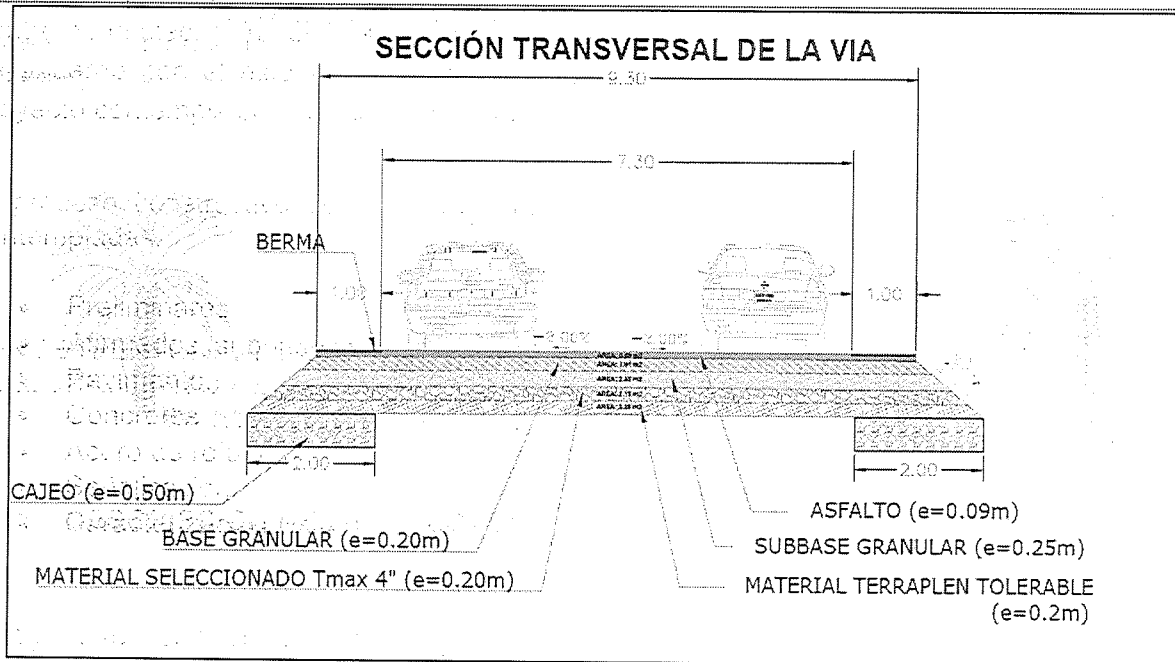
Ilustración 1 Detalle de la sección transversal típica de la intervención Fuente: Archivos del proyecto
