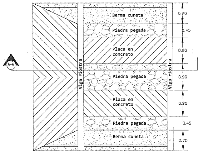
Ilustración 1 Detalle de la Placa Huella
