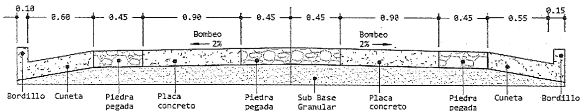
Ilustración 2 Sección Tipo de la Placa Huella
