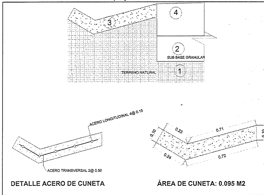
Ilustración 1 Detalle de la estructura de pavimento a construir Fuente: Archivos del proyecto – Diseño de Pavimento
