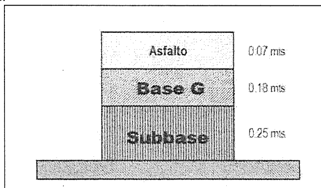
Ilustración 1 Detalle de la estructura de pavimento a construir Fuente: Archivos del proyecto – Diseño de Pavimento Flexible
