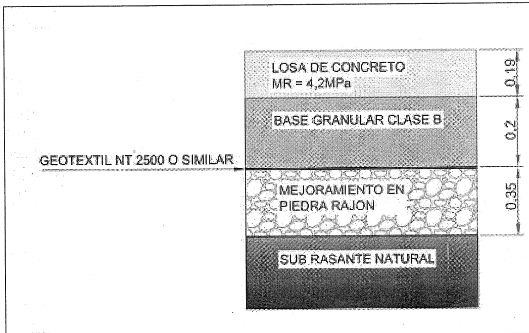
Ilustración 2 Detalle Estructura de pavimento a construir Fuente: Archivos del proyecto – Diseño de Pavimento
