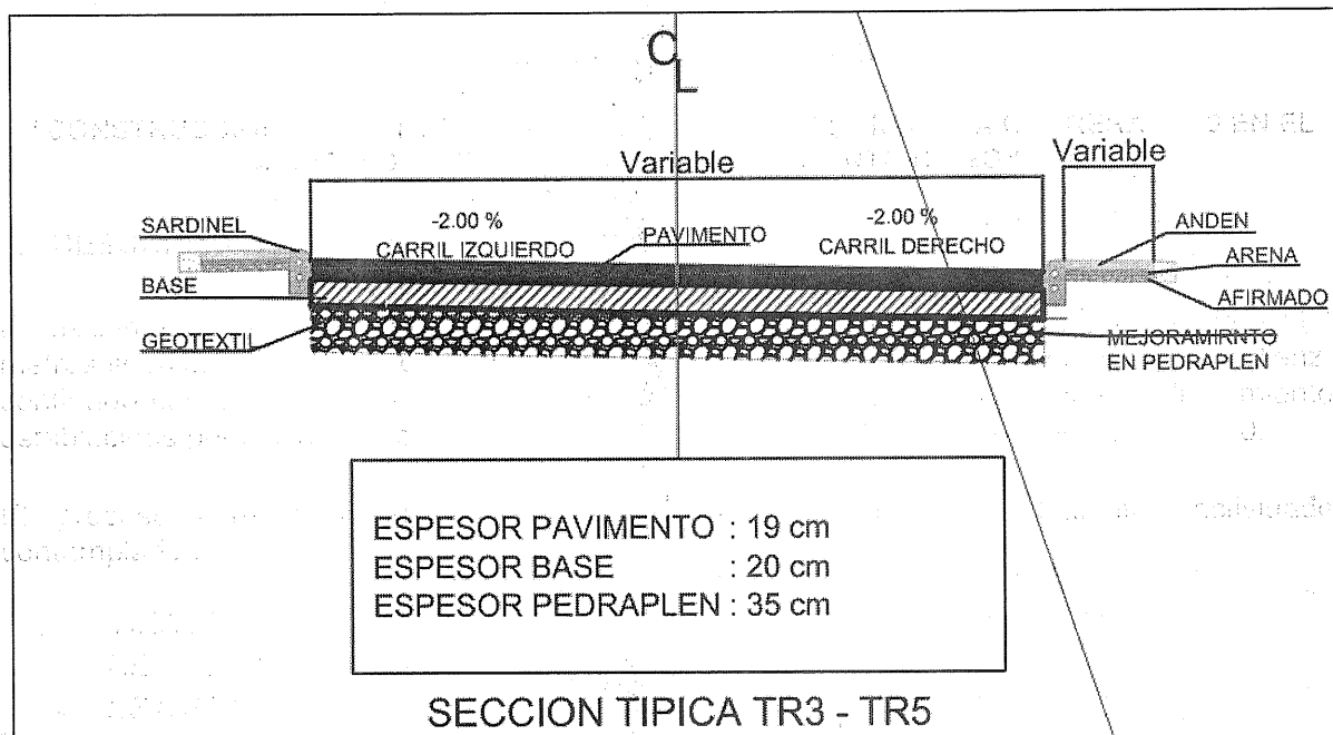
Ilustración 1 Detalle Sección Transversal de la estructura de pavimento a construir Fuente: Archivos del proyecto – Diseño de Pavimento
