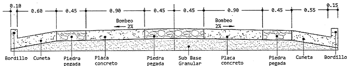
Ilustración 2 Sección Tipo de la Placa Huella Fuente: Archivos del proyecto – Diseño de Estructura Placa Huella
