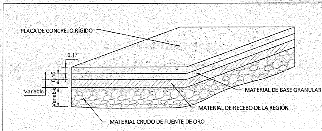
Figura 1. Estructura de pavimento
